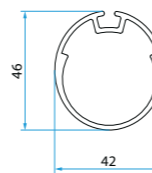
A3505_0508 Adattatori tubo Ovale 42X46
