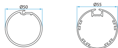
A3505_0517 Adattatori tubo Tondo Ø50 scanalato - Tondo Ø55 Zanzar System
