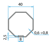
A3505_0502 Adattatori tubo Ottagonale 40 (Graffa interna)
