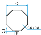
A3505_0501 Adattatori tubo Ottagonale 40 (Graffa esterna)
