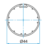
A3505_0515 Adattatori tubo Tondo Filtersun 44
